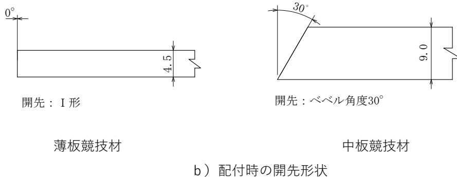
図1 競技用材料の形状および配布時の開先形状
