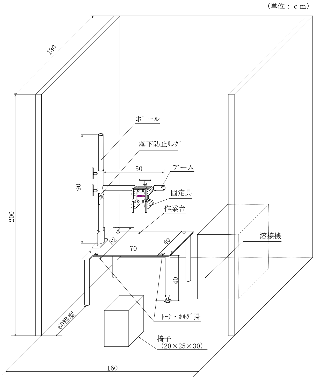
図3 溶接ブース・作業台の概要
