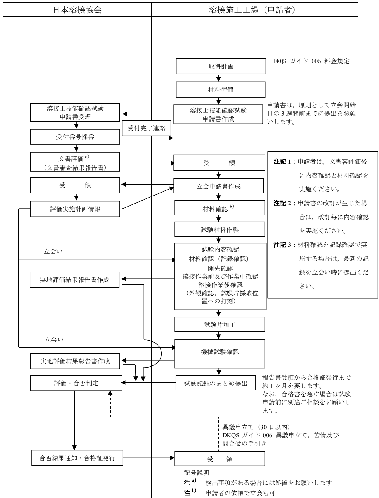
図 I-1-0—溶接士技能確認試験の実施手順概要
