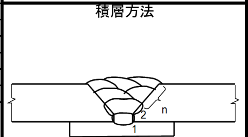
積層方法の例
