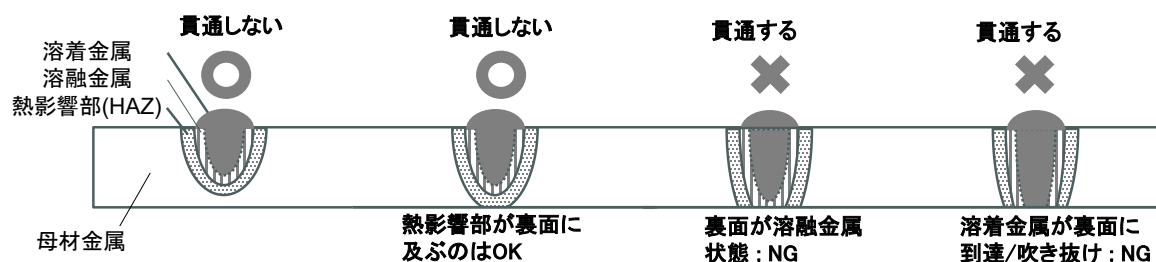
解説図 1—耐圧部材を貫通する溶接及び貫通しない溶接の例
