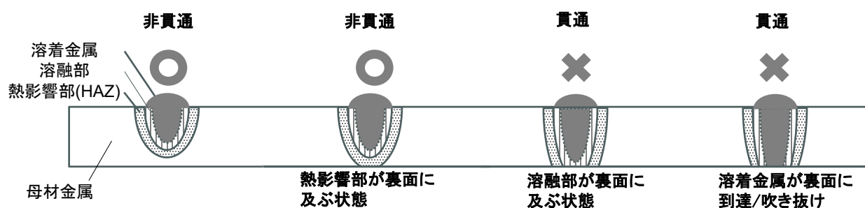
解説図 1 —耐圧部材を貫通した溶接及び貫通していない溶接の例
