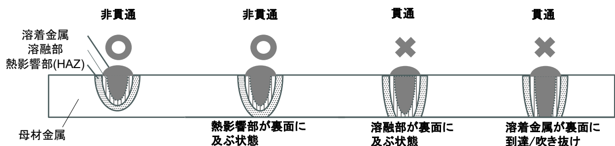
解説図 1—耐圧部材を貫通した溶接及び貫通していない溶接の例
