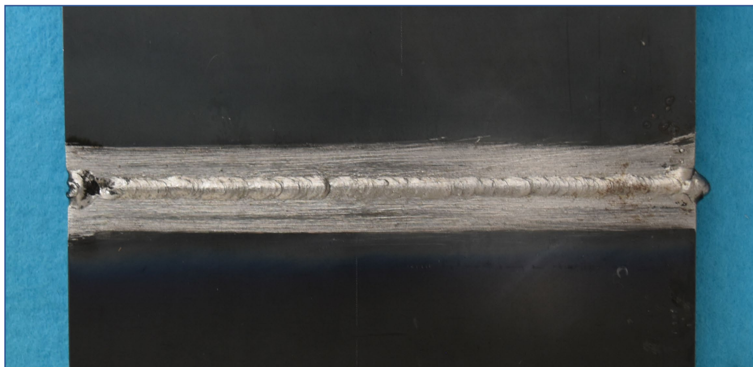
手溶接(薄板)裏面【例 4】
