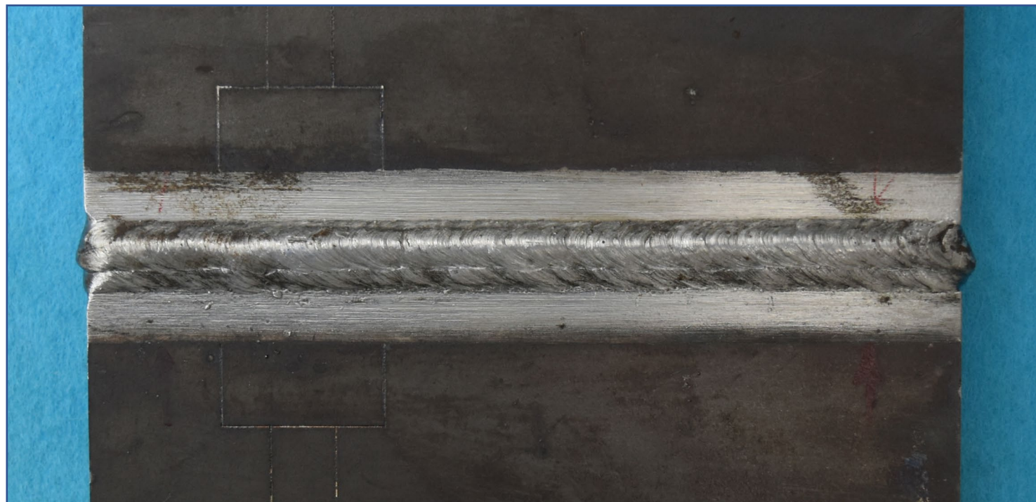
手溶接(中板)表面【例 4】
