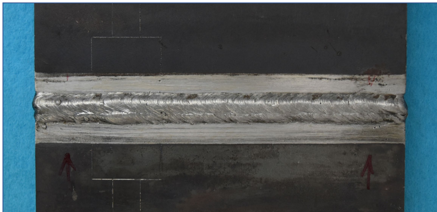
手溶接(中板)表面【例 5】
