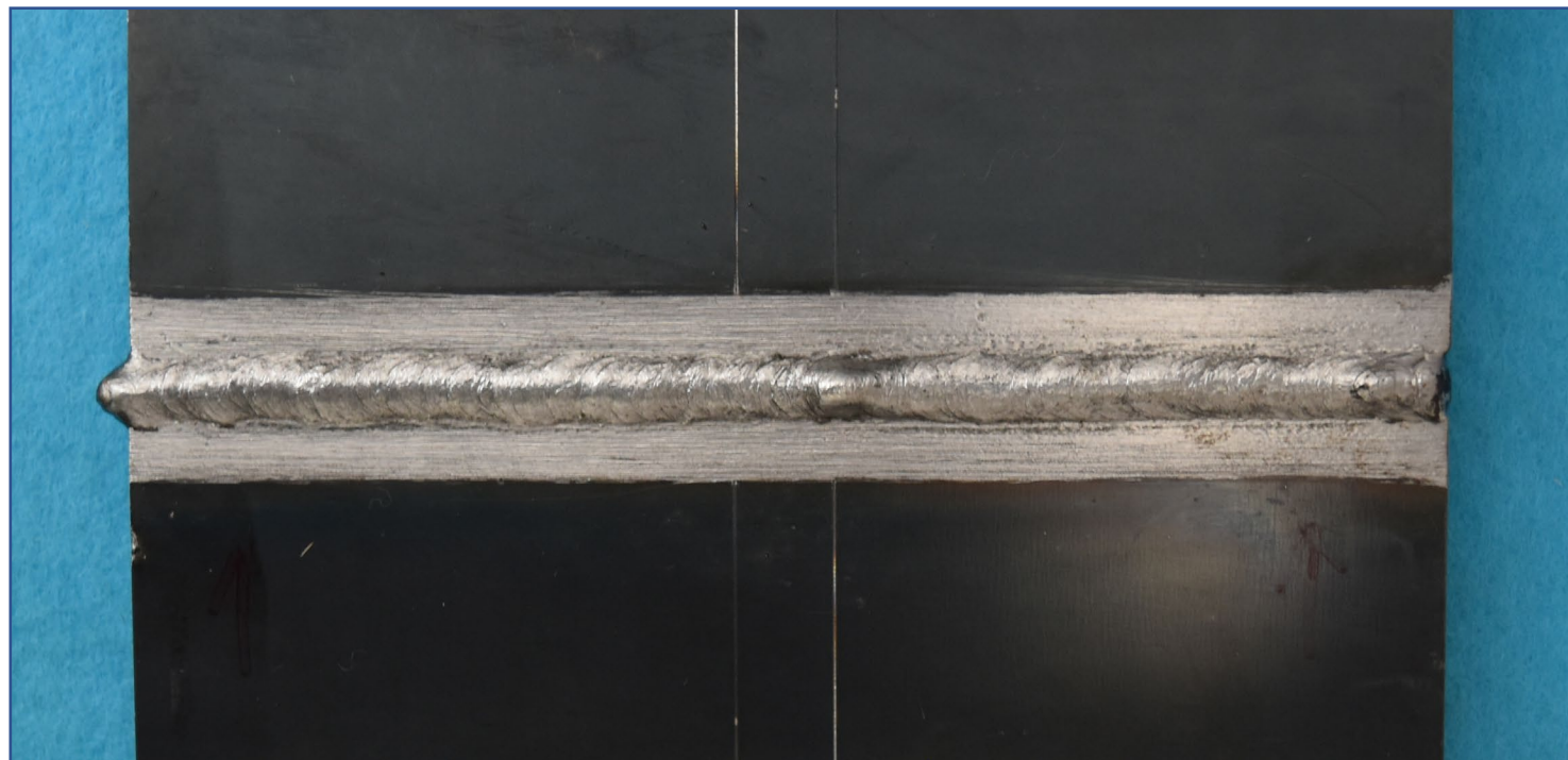
手溶接(薄板)表面【例 4】
