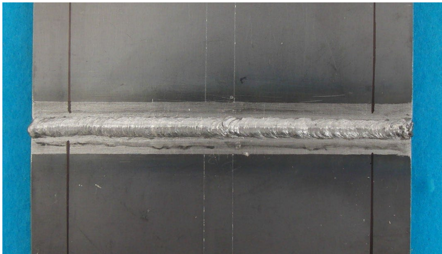
手溶接(薄板)表面【例6】
