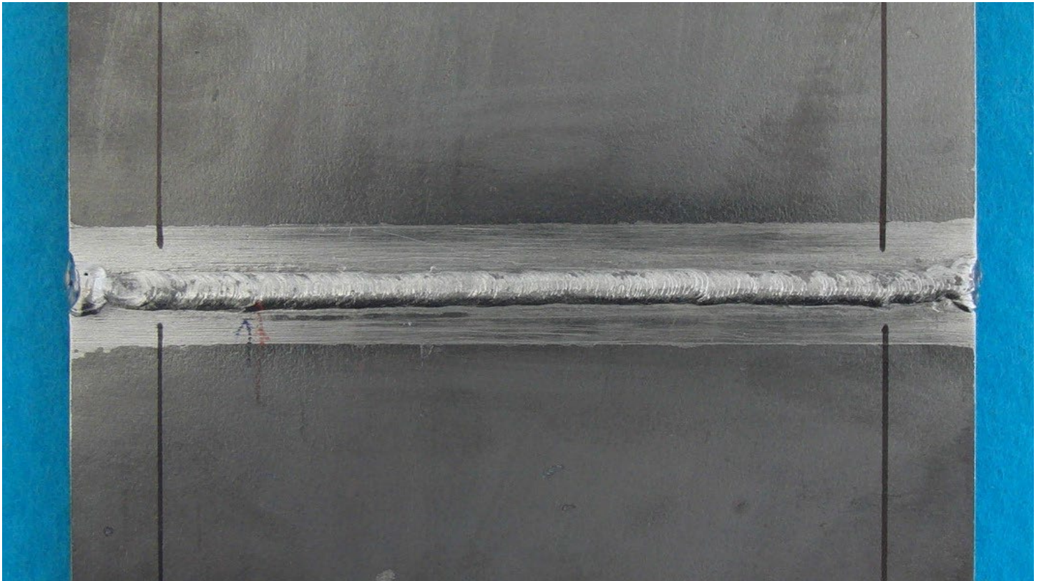
手溶接(中板)裏面【例5】
