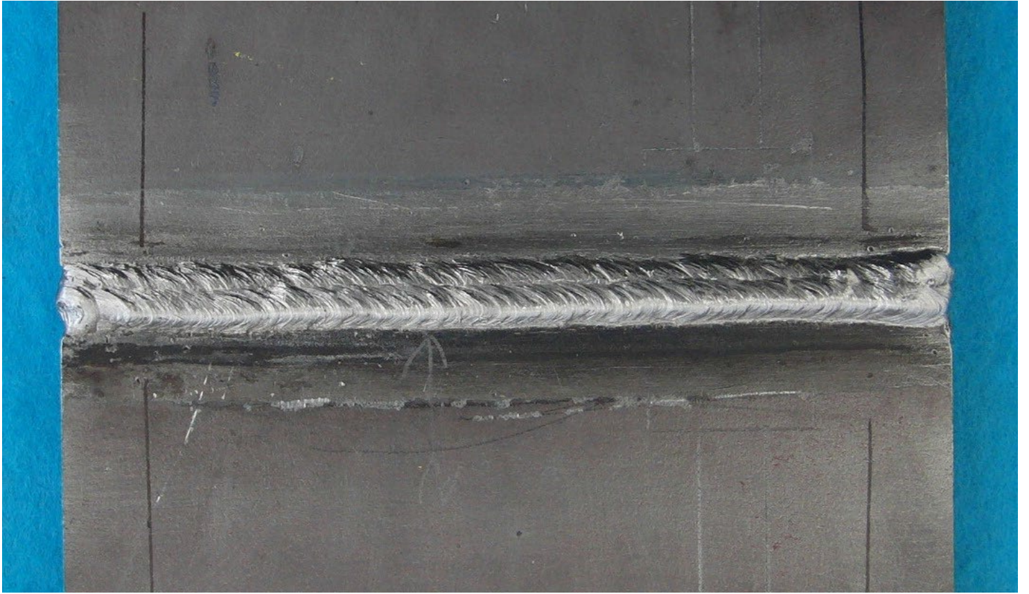
手溶接(中板)表面【例1】
