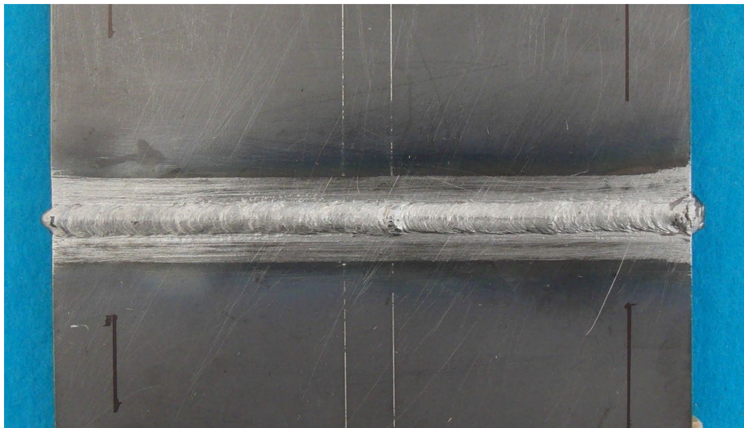
手溶接(薄板)表面【例4】
