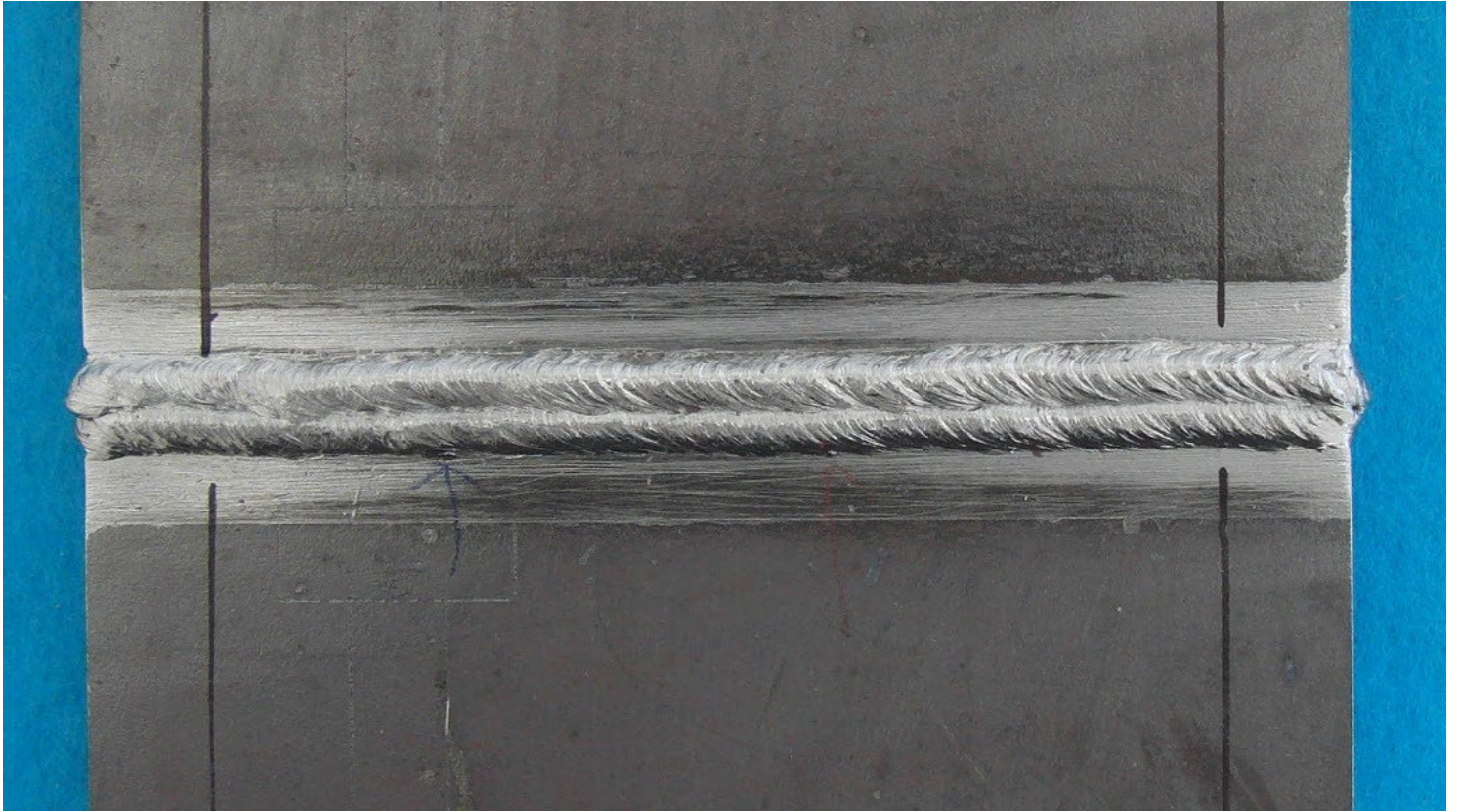
手溶接(中板)表面【例5】
