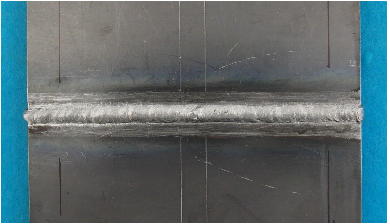
手溶接(薄板)表面【例1】
