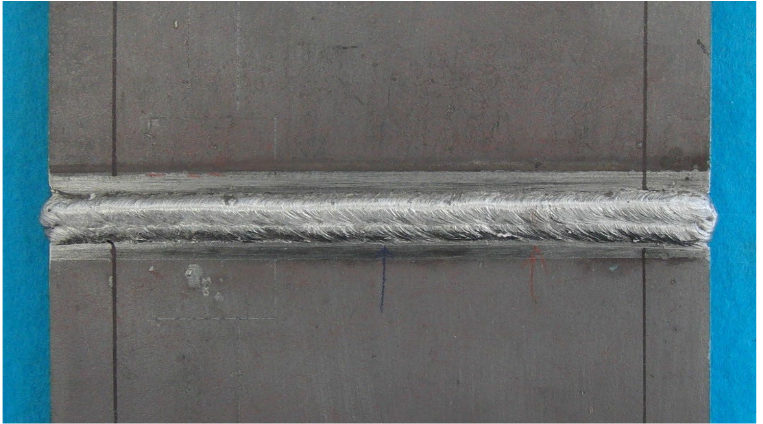
手溶接(中板)表面【例6】
