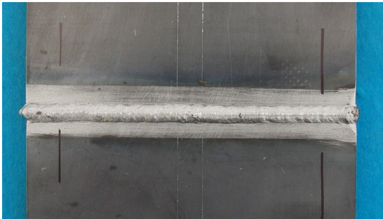
手溶接(薄板)表面【例3】
