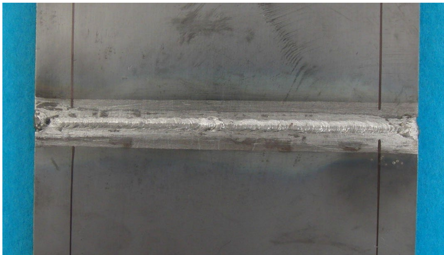
手溶接(薄板)裏面【例6】
