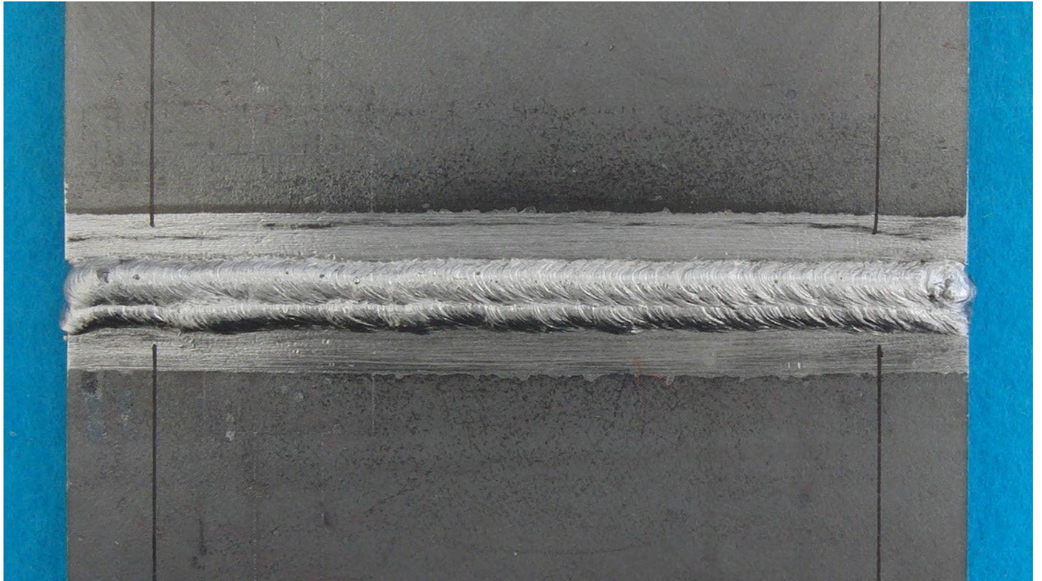
手溶接(中板)表面【例4】
