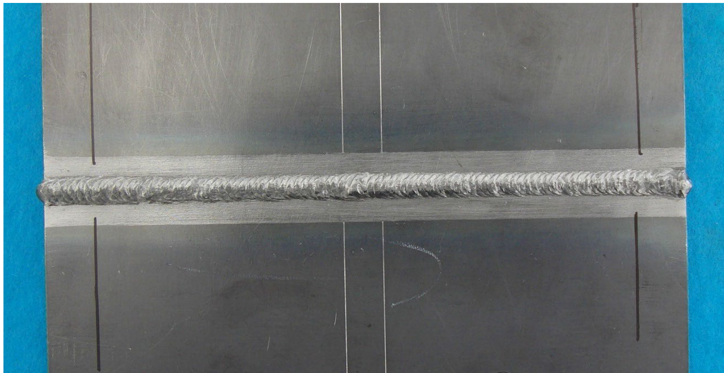
半自動溶接(薄板)表面【例2】
