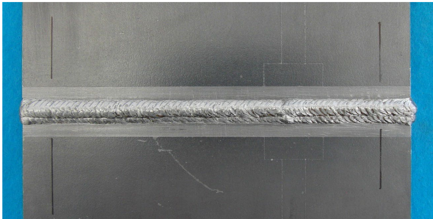
半自動溶接(中板)表面【例6】
