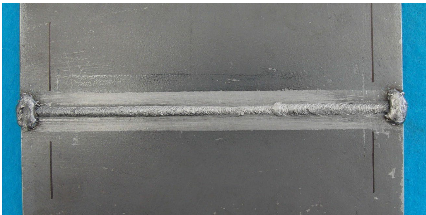
半自動溶接(中板)裏面【例8】
